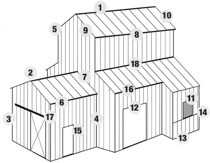
7 - Sidewall
