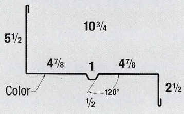
9 - Shadow Rake Trim
