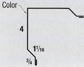
5 - Soffit
