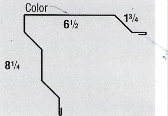
9 - Shadow Rake Trim
